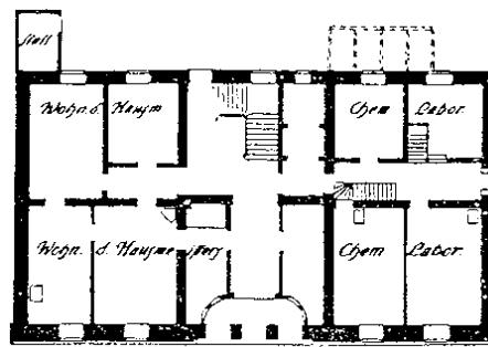
Neues Museum 1830. Erdgeschoß
