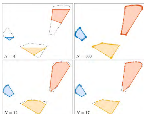
Adaptive Approximation mit der Polygon inflation Methode
