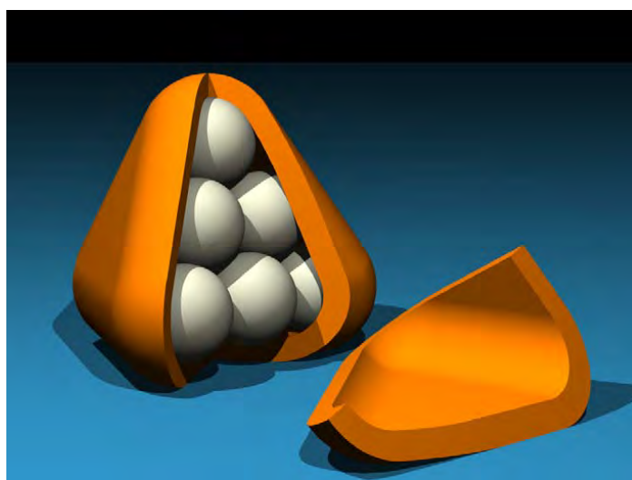
Modell einer Kugelpackung
