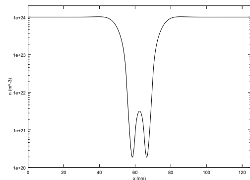
Elektronendichte an einer Resonanttunneldiode im thermischen Gleichgewicht
